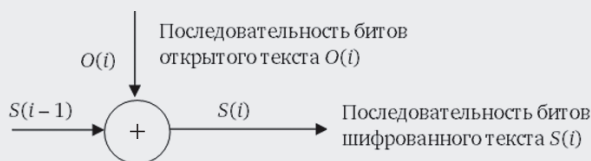
Рис. 3. Схема преобразования закодированного сообщения
