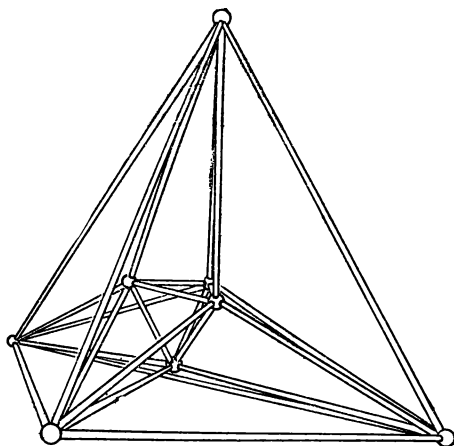
Рис. 171. 16-ячейка.
