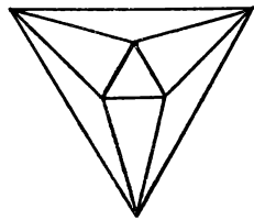
Рис. 155. Октаэдр.
