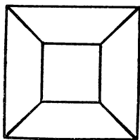
Рис. 154. Куб.
