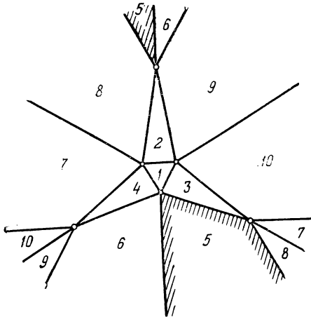
Рис. 168. Икосаэдр.
