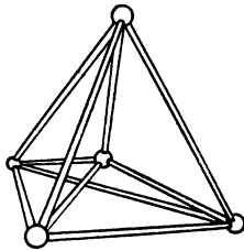
Рис. 169. 5-ячейка.
