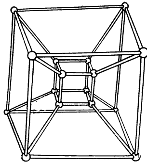
Рис. 170. 8-ячейка.
