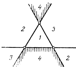
Рис. 165. Октаэдр.
