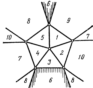
Рис. 163. Икосаэдр.
