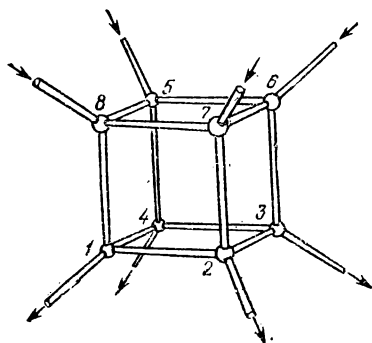
Рис. 174а. 8-ячейка.
