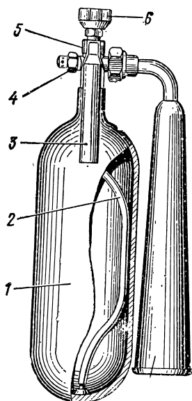
Рис. 43. Устройство углекислотного огнетушителя:
