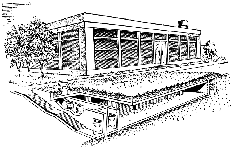
Рис. 4. Отдельно стоящее убежище
