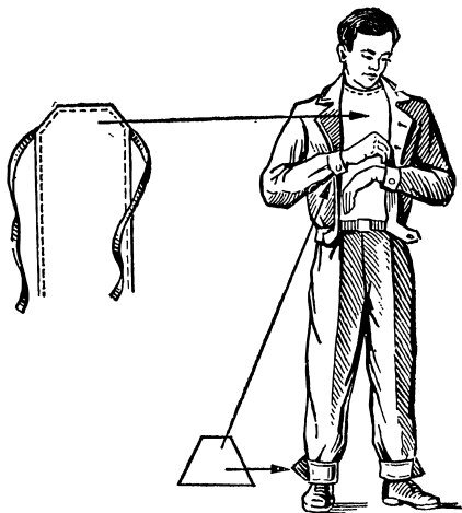
Рис. 23. Герметизация одежды
