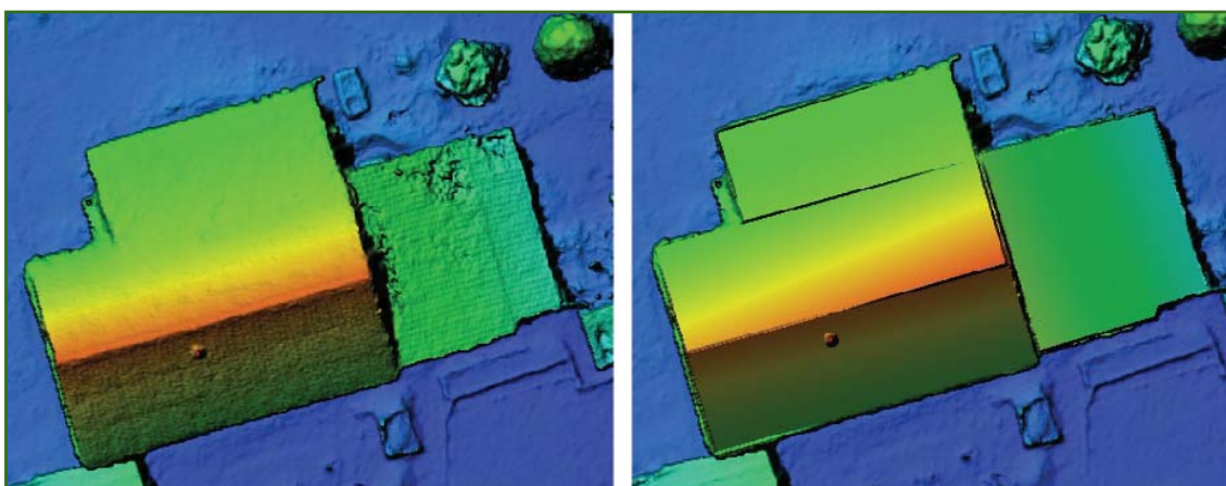
Рис. 4 Редактирование участка наклонной крыши методом аппроксимирующей плоскости: участок крыши до сглаживания (слева), результат сглаживания (справа)
