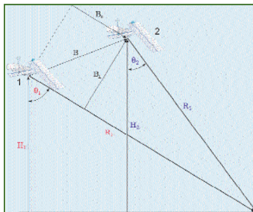
H_1 и H_2 — высота радиолокатора; R_1 и R_2 — дальности (пути зондирующей волны); \theta_1 и \theta_2 — углы между дальностью и высотой; B_1 и B_2 — перпендикулярная и параллельная составляющие базовой линии B
