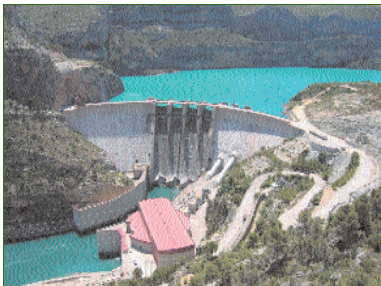
Рис. 3 Наблюдения за деформациями плотин
