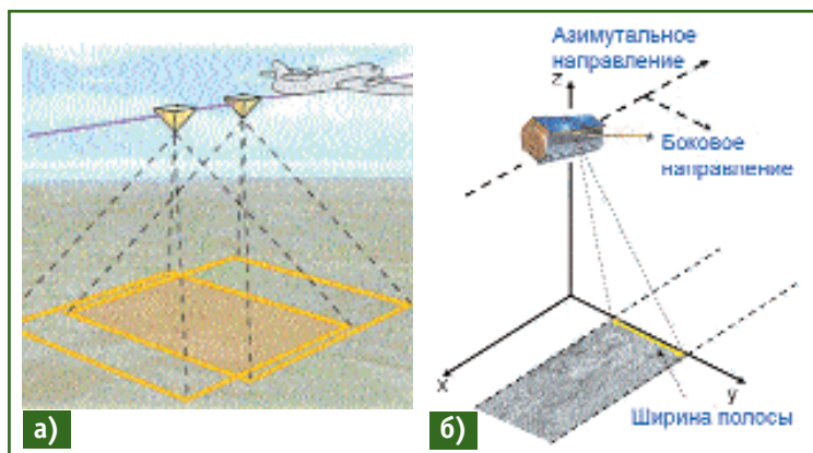
Рис. 4 Геометрия съемки: а) центральная проекция; б) боковая съемка
