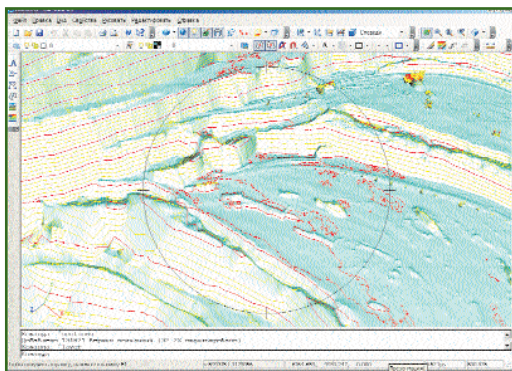
Рис. 4 Модель участка карьера Качканарского ГОК с построенными изолиниями в программе GK3DModeller
