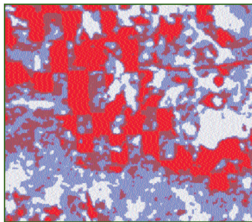
Рис. 5 Метод Division*
