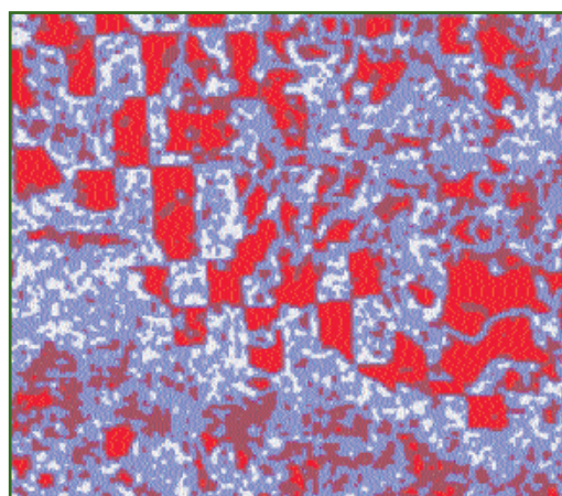
Рис. 6 Метод PCA*
