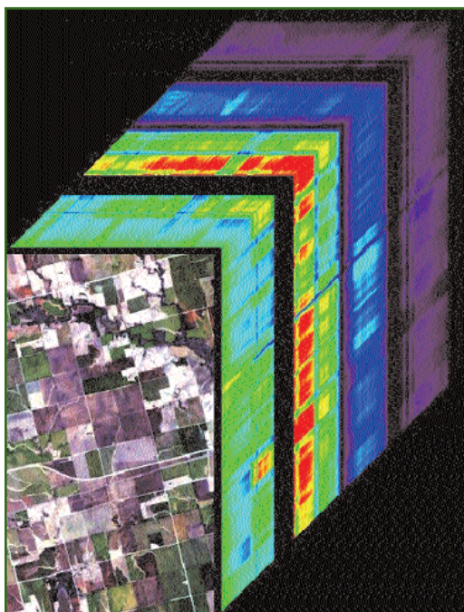
Рис. 1 «Гиперспектральный куб» для фрагмента снимка HYPERION
