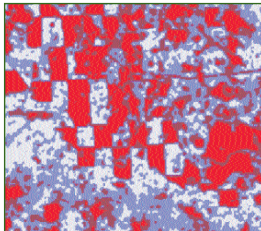
Рис. 4 Метод Subtraction*
