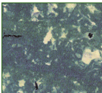
Рис. 2 Фрагмент снимка со спутника Landsat-5 (4 апреля 1986 г.)
