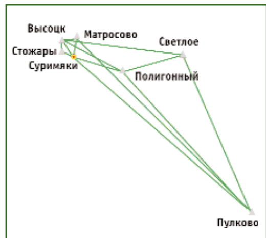
Рис. 4 Схема геодезической основы в районе работ
