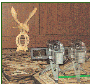
Рис. 6 Стереосъемка неподвижного объекта одной камерой с двух точек
