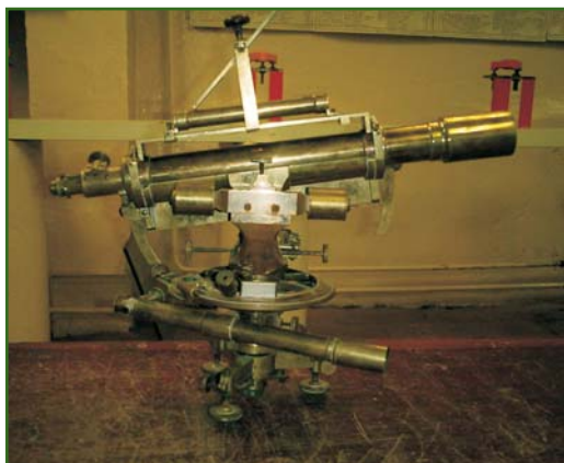
Рис. 2 Нивелир-теодолит середины XIX века (Kern, Швейцария)
