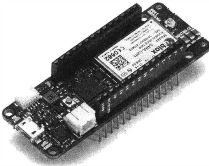
Рис. 2.10. Плата Arduino MKR GSM 1400
