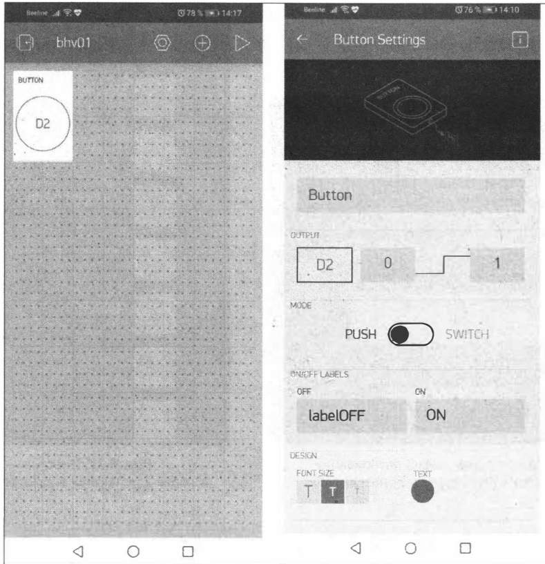
Рис. 5.78. Виджет Button
