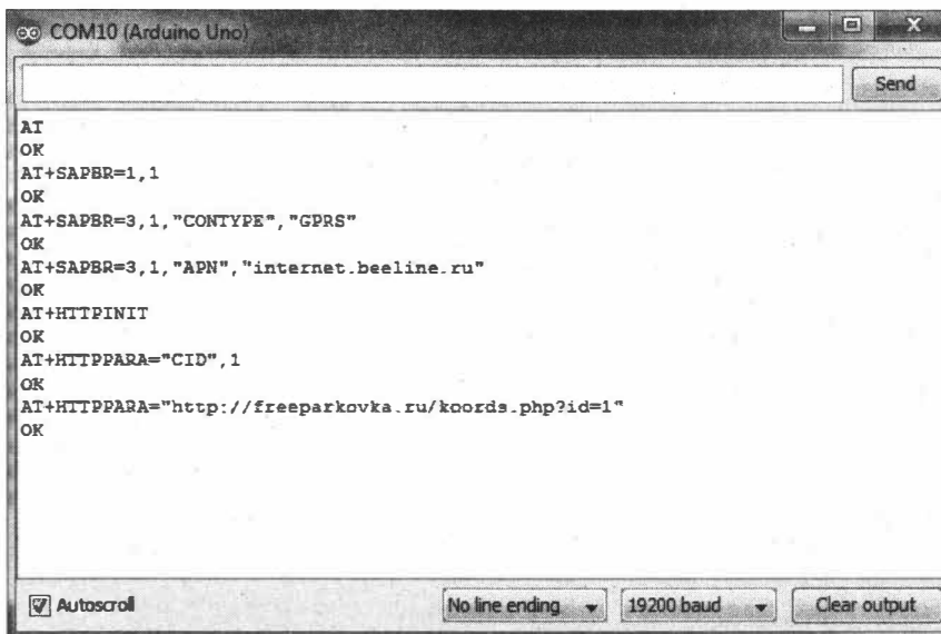
Рис. 3.34. Отправка AT-команд на GSM/GPRS Shield SIM900 из последовательного порта
