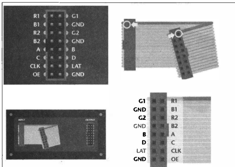
Рис. 6.7. Подключение RGB-матрицы 64×32
