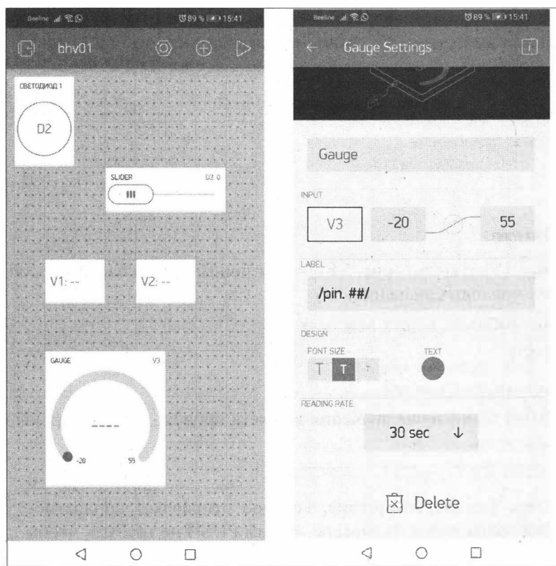
Рис. 5.81. Виджет Gauge
