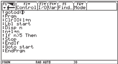
Рис. 11.22. Пример применения оператора Goto безусловного перехода
