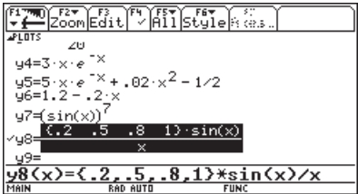
Рис. 9.76. Задание функции y8 с параметром в виде списка
