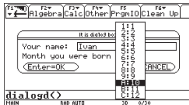
Рис. 11.28. Диалоговое окно ввода, создаваемое при исполнении программы dialogd
