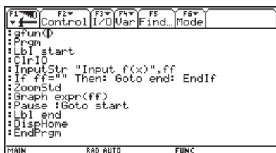
Рис. 11.32. Программа построения графика выражения с его интерактивным вводом
