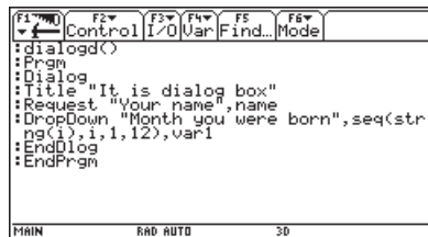
Рис. 11.27. Программа dialogd, демонстрирующая создание диалогового окна
