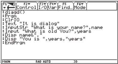
Рис. 11.24. Пример простой диалоговой программы diagd
