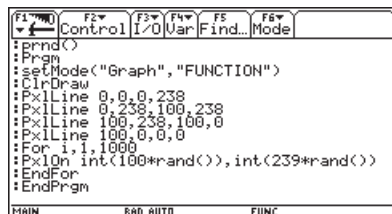
Рис. 11.34. Программа построения случайных точек в окне графики
