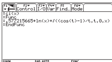
Рис. 11.11. Функция вычисления интегрального косинуса
