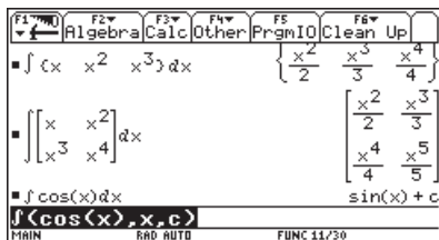
Рис. 8.28. Дополнительные примеры интегрирования
