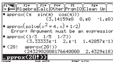
Рис. 8.13. Примеры применения функции approx
