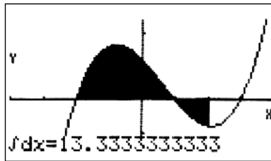
Рис. 6.7. График заданной функции с иллюстрацией вычисления определенного интеграла
