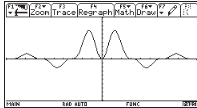
Рис. 11.33 График выражения 10 \cdot \sin(x)^3/x , введенного в окне ввода/вывода
