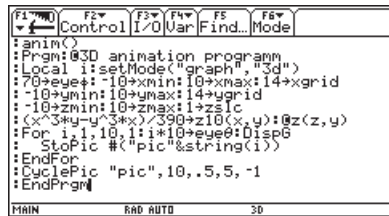
Рис. 11.36. Программа анимации поверхности
