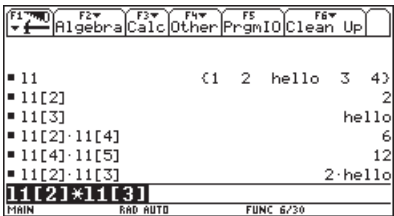
Рис. 10.4. Выполнение операций над списком l1 в окне Nome
