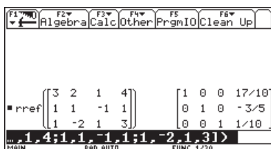
Рис. 8.7. Пример решения системы из трех уравнений функцией rref
