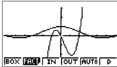
Рис. 6.6. Графики двух функций в декартовой системе координат
