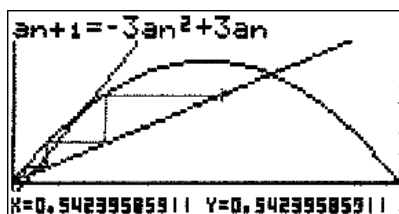
Рис. 6.25. Начало сходящегося процесса рекурсии
