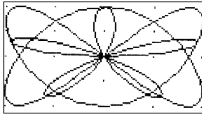
Рис. 6.11. Графики параметрически заданной функции и функции в полярной системе координат (пятиконечная «роза»)
