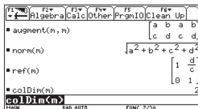
Рис. 10.13. Демонстрация работы функций augment, notm, ref и colDim
