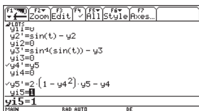
Рис. 9.67. Задание уравнений Ван-дер-Поля
