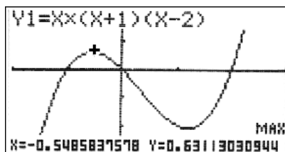
Рис. 6.13. Нахождение максимума функции
