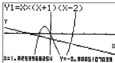
Рис. 6.9. Пример построения перпендикуляра к точке графика
