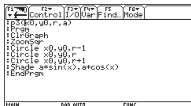
Рис. 11.9. Процедура со списком параметров
