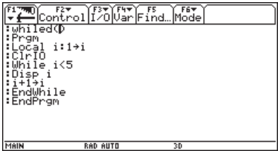
Рис. 11.21. Пример задания цикла While-End
