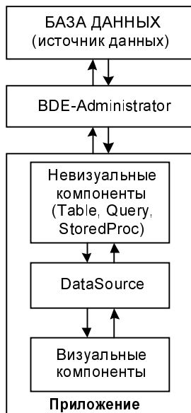
Рис. 7.1. Схема взаимодействия программ с данными
