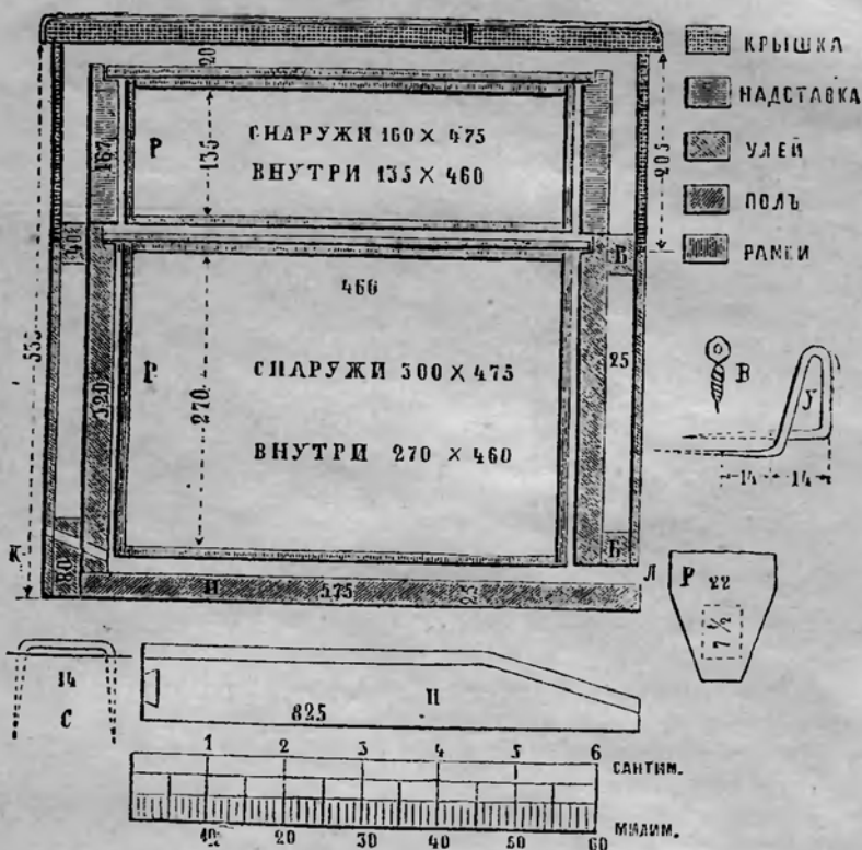
Рис. 16. Чертеж американскаго улья Дадана (улей Дадана см. рис. 17 и 18)—Цифры показывают количество миллиметровъ въ частяхъ улья. Подъ буквою П означенъ подставной полъ съ прилетною доскою. Подъ буквою Р конецъ рамки, У—угольникъ, С—скобочки, служащія раздѣлителями между рамками.
