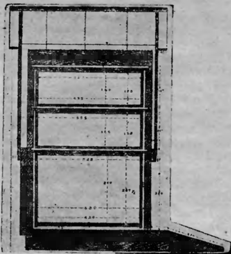
Рис. 21. Продольный разрѣзъ улья Дадана-Блатта. (1/15 натуральной величины).
