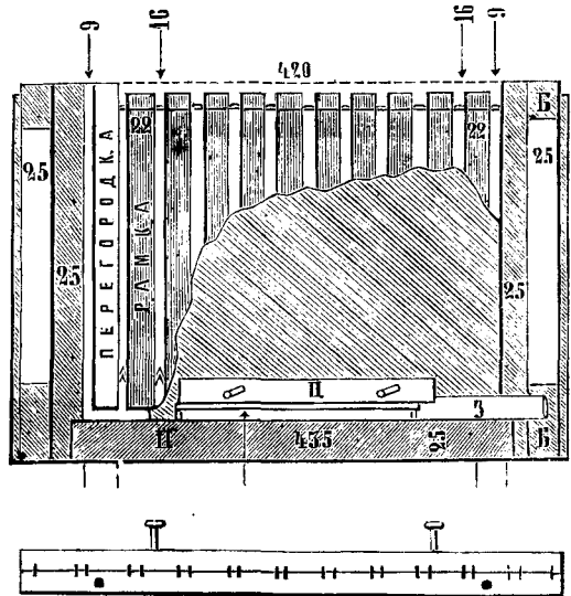
Форма для вбиванія раздѣлителей.
