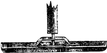
Прикрѣпленіе оси медогонки.
