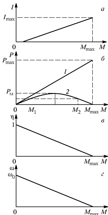
Рис. 122. Зависимость тока в обмотке якоря (а), полной и полезной мощности (б), КПД (в) и угловой скорости якоря (з) от момента внешних сил
