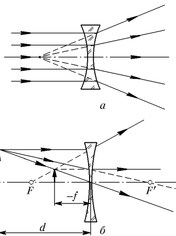
Рис. 241. Рассеивающая линза
