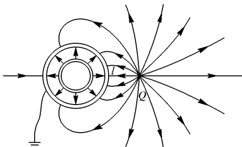
Рис. 46. Сферический конденсатор во внешнем электрическом поле
