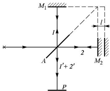
Рис. 198. Схема интерферометра Майкельсона
