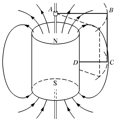
Рис. 116. Униполярный индуктор
