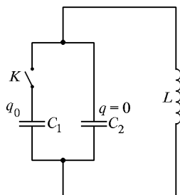
Рис. 164. Электрическая цепь, для которой не выполняются условия квазистационарности
