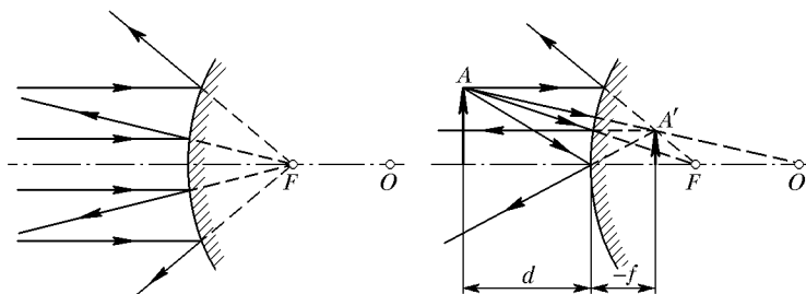
Рис. 238. Выпуклое зеркало
