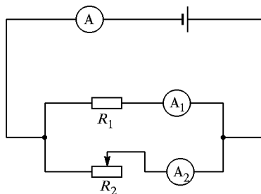
Рис. 78. К исследованию изменений показаний амперметров
