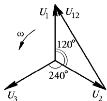
Рис. 150. Векторная диаграмма фазных напряжений при соединении звездой
