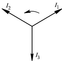
Рис. 151. Векторная диаграмма токов в соединении звездой при одинаковых нагрузках
