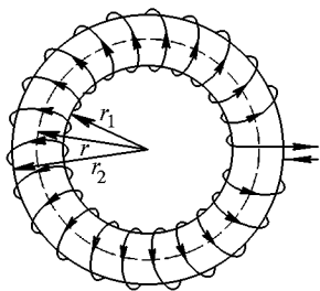
Рис. 97. Тороидальная катушка
