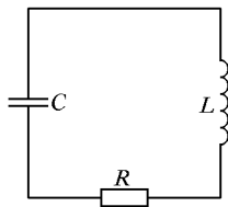
Рис. 160. Колебательный контур с сопротивлением
