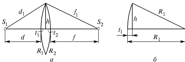
Рис. 230. К выводу формулы тонкой линзы
