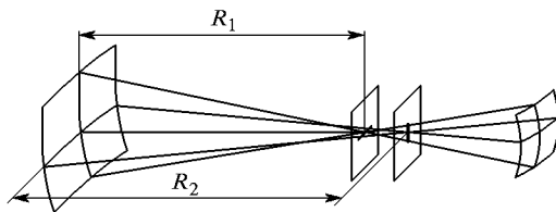
Рис. 235. Астигматический пучок лучей
