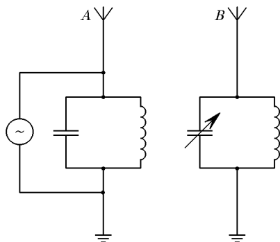
Рис. 190. Схема радиосвязи
