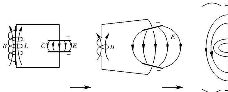
Рис. 176. Переход от колебательного контура к открытому вибратору
