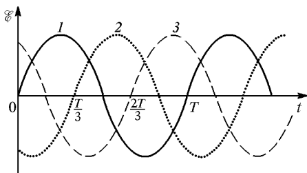
Рис. 147. Графики ЭДС, сдвинутых по фазе на 120^\circ
