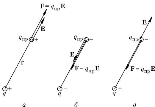
Рис. 6. Напряженность \mathbf{E} поля, создаваемого зарядом q , и сила \mathbf{F} , действующая на пробный заряд q_{\text{пр}}
