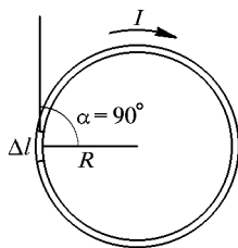
Рис. 92. К вычислению магнитного поля кругового тока
