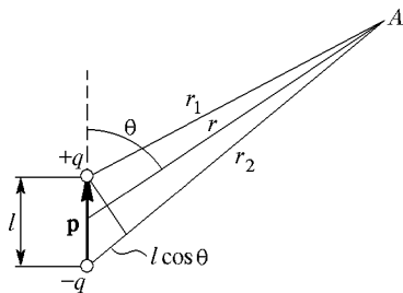
Рис. 22. Вычисление потенциала диполя в точке А
