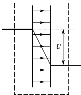
Рис. 49. Электрическое поле заряженного плоского конденсатора
