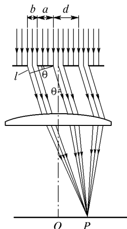
Рис. 211. К объяснению действия дифракционной решетки
