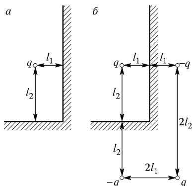
Рис. 34. Электрическое поле внутри двугранного угла ( a ) совпадает с полем четырех зарядов ( b )
