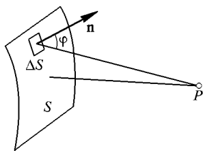
Рис. 199. К расчету дифракции на основе принципа Гюйгенса—Френеля
