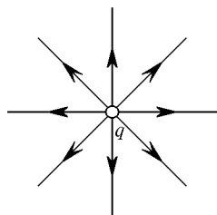
Рис. 179. Поле неподвижного точечного заряда
