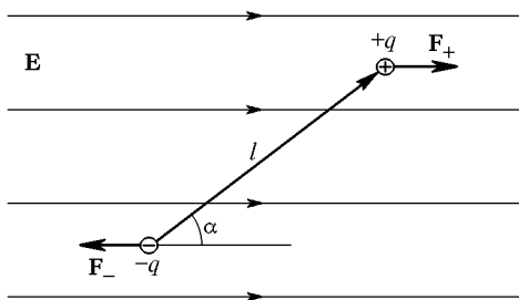
Рис. 36. Силы, действующие на диполь в однородном электрическом поле
