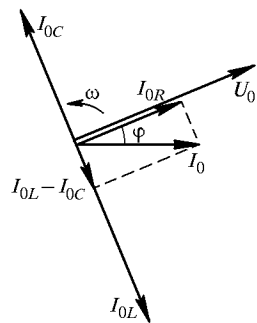
Рис. 142. Векторная диаграмма для параллельной RLC -цепи
