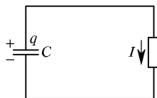
Рис. 133. При разрядке конденсатора значение силы тока I связано с зарядом верхней пластины соотношением I = -dq/dt
