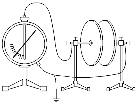
Рис. 43. Емкость конденсатора зависит от расстояния между пластинами
