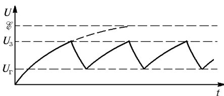
Рис. 175. Зависимость напряжения на конденсаторе от времени
