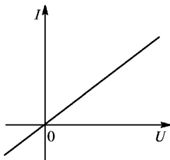
Рис. 59. Вольт-амперная характеристика проводника, подчиняющегося закону Ома
