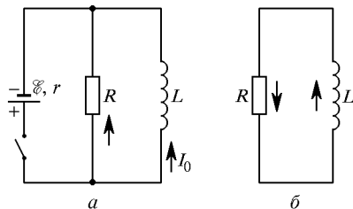
Рис. 123. Электрическая цепь для изучения магнитной энергии тока
