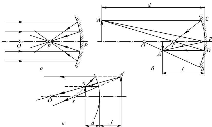
Рис. 237. Вогнутое зеркало
