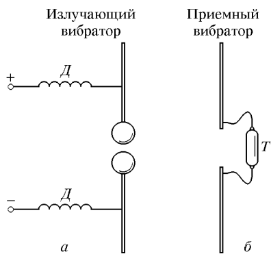
Рис. 178. Вибратор Герца
