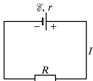
Рис. 76. Простейшая замкнутая цепь с источником тока
