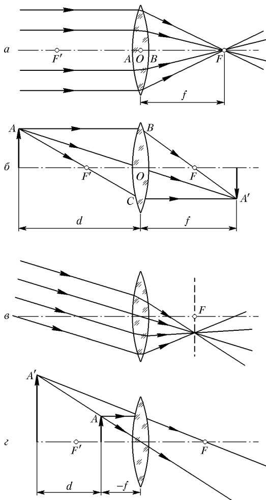
Рис. 240. Собирающая линза
