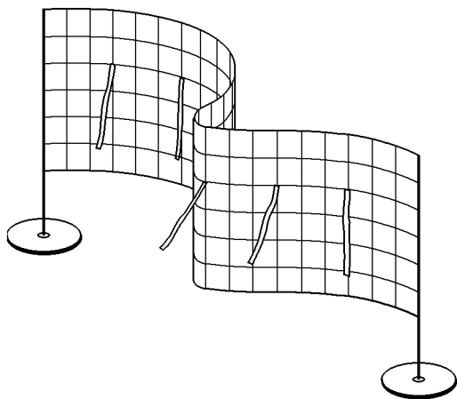
Рис. 28. Листочки сильнее отклоняются на внутренних участках сетки
