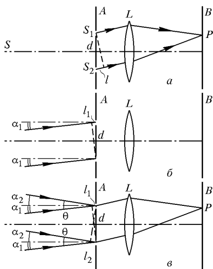
Рис. 216. К объяснению принципа действия звездного интерферометра
