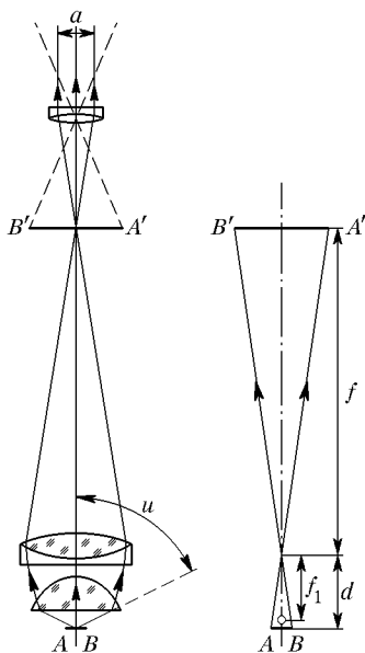
Рис. 246. Микроскоп
