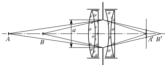
Рис. 242. Фотоаппарат
