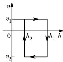
Рис. 173. Фазовая диаграмма релаксационных колебаний, показанных на рис. 172
