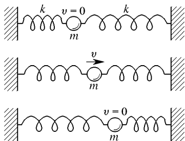
Рис. 163. Механическая аналогия для электрической цепи, показанной на рис. 162
