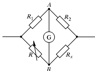
Рис. 71. Мост Уитстона
