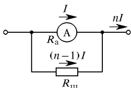
Рис. 68. Шунтирование амперметра
