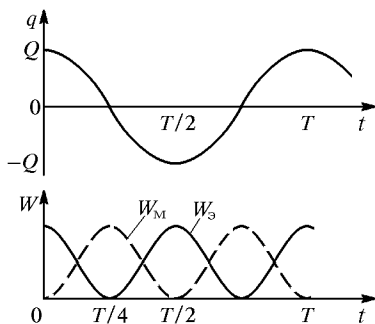
Рис. 159. Графики зависимости от времени заряда конденсатора q , энергии W_э электрического поля конденсатора и энергии W_м магнитного поля в катушке
