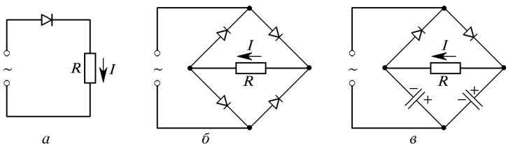
Рис. 146. Схемы выпрямителей: однопериодного (а), двухпериодного (б) и с удвоением напряжения (в)
