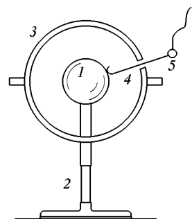
Рис. 26. Опыт Кавендиша
