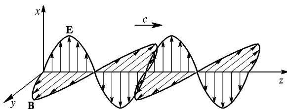
Рис. 185. Электрическое и магнитное поля в бегущей линейно поляризованной волне
