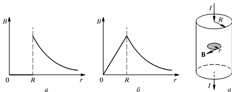
Рис. 98. Магнитное поле прямого тока, текущего по поверхности цилиндрического проводника (а), по всему сечению (б); к расчету магнитного поля внутри проводника (в)
