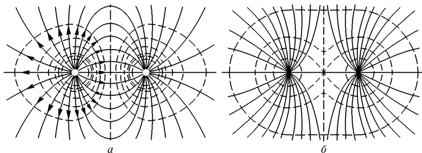
Рис. 14. Линии напряженности и эквипотенциальные поверхности поля разноименных (а) и одноименных (б) одинаковых по модулю точечных зарядов
