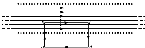
Рис. 96. Контур для применения теоремы о циркуляции
