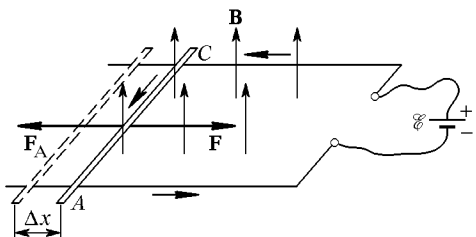
Рис. 121. К энергетическим превращениям при электромагнитной индукции
