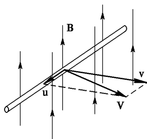
Рис. 114. Скорость носителя заряда в движущемся проводнике
