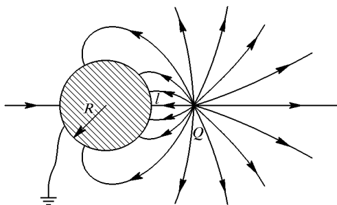
Рис. 47. Поле точечного заряда вблизи заземленного проводящего шара
