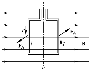
Рис. 101. К выводу выражения для силы Ампера
