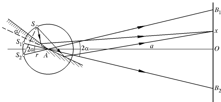
Рис. 197. Изображения реального источника света в плоских зеркалах, расположенных под малым углом друг к другу
