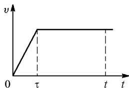
Рис. 180. График скорости заряда
