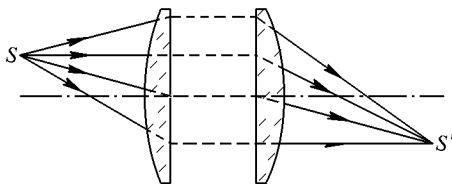
Рис. 236. Образование изображения в оптической системе
