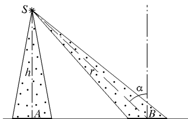
Рис. 252. Освещенность поверхности, создаваемая точечным источником
