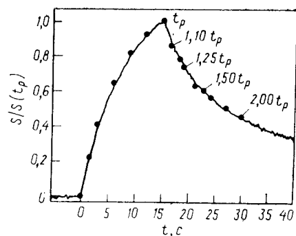
Рис. 3.45. Зависимость сигнала ЭПР от времени для раствора диэтилфумарата (7,5 ммоль/л) Продолжительность импульса тока t_p = 15 с, I = 0,21 мА [201]
