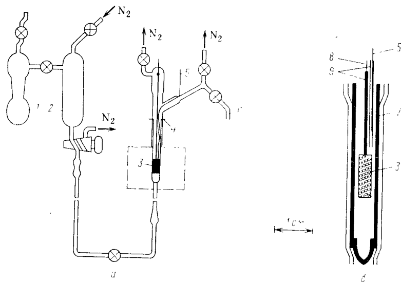
Рис. 3.43. Схема установки для электрохимического генерирования радикалов в полости спектрометра ЭПР:
