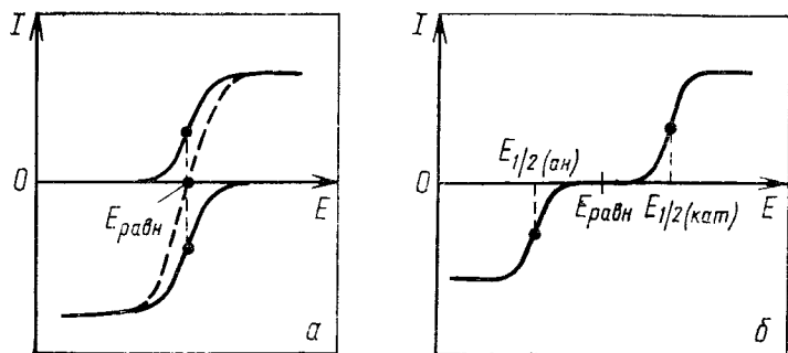
Рис. 2.6. Кривые ток — потенциал быстрой (а) и медленной (б) систем
