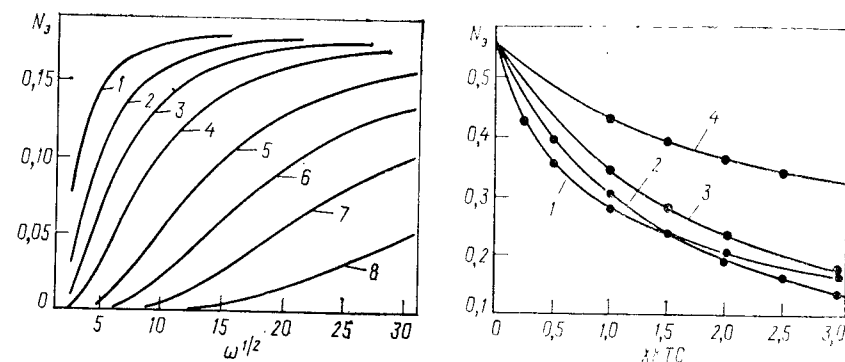
Рис. 3.26. Рабочие кривые в методе вольтамперометрии с вращающимся дисковым электродом с кольцом для механизма ECE при константах скорости стадии С, равных 0,2 (1), 0,5 (2), 1 (3), 2 (4), 5 (5), 10 (6), 20 (7) и 50 (8) \text{с}^{-1} . При k=0 N_3=0,184
