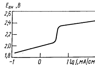
Рис. 14.1. Зависимость анодного потенциала от логарифма плотности тока при электролизе 0,5 \text{ М} водного раствора ацетата натрия [14]
