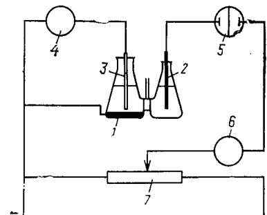
Рис. 5.13. Схема установки для восстановления при постоянном потенциале [43]:
