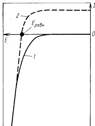
Рис. 2.9. Окисление серебряного электрода в ацетонитриле, содержащем \text{LiClO}_4 ( 10^{-1} моль/л):
