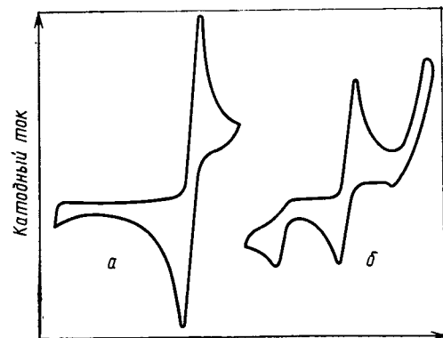
Рис. 6.3. Вольтамперные кривые восстановления 9,10-дифенилантрацена на платиновом микроэлектроде в ДМФА, содержащем n\text{-Bu}_4\text{NClO}_4 (непрерывная линейная развертка потенциала, 4,7 В/с [125]):
