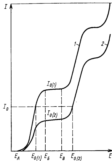
Рис. 5.1. Схематичное изображение соотношения между током и потенциалом рабочего электрода до электролиза (1) и в ходе электролиза (2) в растворе, содержащем соединение с двумя группами, восстанавливающимися при различных потенциалах:
