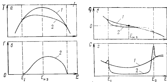
Рис. 2.24. Зависимость пограничного натяжения \gamma (а), поверхностной концентрации \Gamma нейтрального адсорбированного вещества (б), плотности заряда q (в) и дифференциальной емкости C (г) электрода от потенциала:
