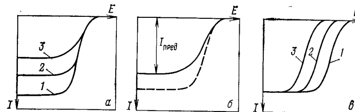
Рис. 2.19. Кривые ток — потенциал при окислении ароматического амина в присутствии кислоты:
