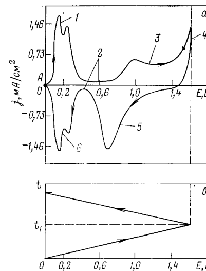
Рис. 2.28. Циклическая вольтамперограмма (а), соответствующая треугольному изменению потенциала (б), на платиновом электроде в водном 2,3 М растворе H_2SO_4 при 25 °С (электрод сравнения H_2/H^+ ; скорость разворота потенциала 0,5 В/с): 1 — окисление адсорбированного водорода; 2 — область двойного слоя; 3 — образование оксида; 4 — выделение кислорода; 5 — восстановление оксида; 6 — восстановление H^+ и адсорбция водорода.
