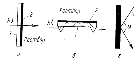
Рис. 3.33. Электроды для спектродэлектрохимии:
