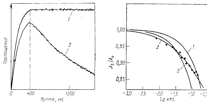
Рис. 3.40. Кривые поглощение — время для спектроэлектрохимического генерирования анион-радикалов перилена в ДМФА при 570 нм [192]:
