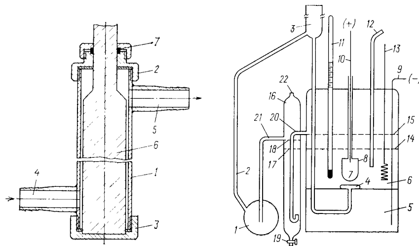
Рис. 5.7. Поперечный разрез концентрической капиллярной щелевой ячейки [70a]:
