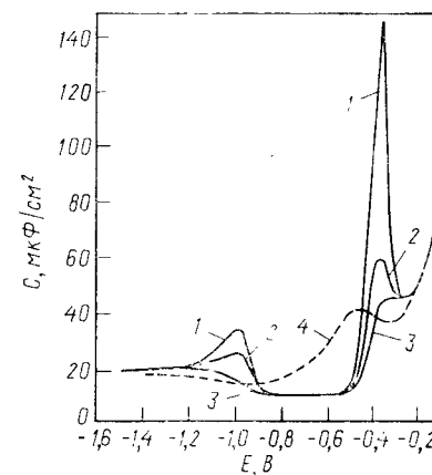
Рис. 2.26. Зависимость дифференциальной емкости висящей ртутной капли при 25 °С в 1 М водном растворе \text{KCl} , содержащем 10^{-2} моль/л n -пентилового спирта, от потенциала при частоте (электрод сравнения — насыщенный каломельный электрод):
