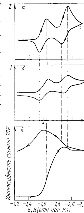
Рис. 3.44. Циклические вольтамперограммы циклооктатетраена в ГМФТА, снятые на электроде в виде висющей ртутной капли (а) и в ячейке для ЭПР на амальгамированном золотом электроде площадью 15 \text{ см}^2 (б), и зависимость интенсивности сигнала ЭПР от потенциала (в), записанная одновременно с кривой (б) [204]
