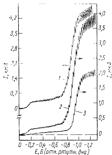
Рис. 3.19. Полярограммы биантрона (1 ммоль/л) в водном феноле [75,4 % (масс.)], содержащем AcONa (0,5 моль/л), при температурах (в °C), равных 60,5 (1), 48,5 (2) и 15,5 (3). Потенциалы приведены относительно ртутного диа [110]
