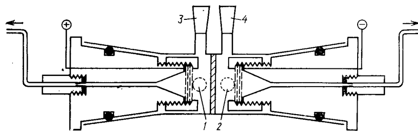
Рис. 5.9. Ячейка непрерывного действия с пористыми электродами [73]: 1, 2 — отверстия для подачи электролита; 3, 4 — отверстия для электрода сравнения
