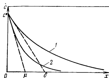
Рис. 2.18. Зависимость концентрации частицы B_1 от расстояния x до поверхности плоского электрода:
