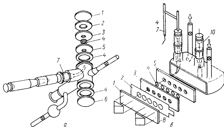
Рис. 3.34. Спектроэлектрохимические ячейки, используемые в спектроскопии пропускания [163] (а) и в спектроскопии внутреннего отражения [172] (б):
