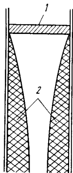
Рис. 3.42. Схема цилиндрической ячейки для спектроскопии ЭПР:
