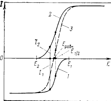
Рис. 2.5. Кривые ток — потенциал для фенотиазина (1), его катион-радикала (2) и их смеси (3)
