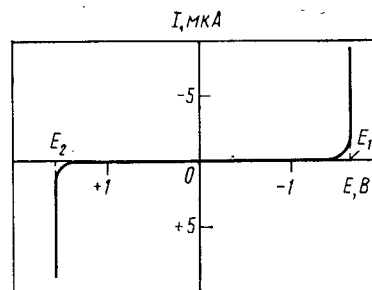
Рис. 2.10. Область электроактивности в растворе \text{Et}_4\text{NClO}_4 ( 10^{-1} моль/л) в нитробензоле на полированном платиновом вращающемся дисковом электроде (электрод сравнения \text{Ag}/\text{AgClO}_4 , 5 \cdot 10^{-3} моль/л) [7]
