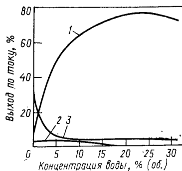
Рис. 6.2. Влияние добавок воды на выход по току 1,4-дигидронафталина (1), 1,2-дигидронафталина (2) и тетралина (3) при электровосстановлении нафталина в ацетонитриле, содержащем n -толуолсульфонат тетраэтиламмония [76]
