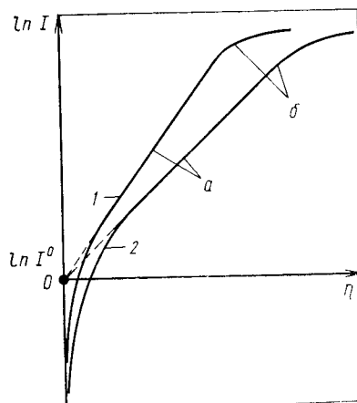
Рис. 2.13. Зависимость тока от перенапряжения \eta для анодной (1) и катодной (2) реакций в системе А/В при \alpha \neq 0,5 : а — область, в которой выполняется тафелевская зависимость; б — области, в которых токи лимитируются скоростью массопереноса
