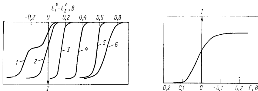
Рис. 2.15. Кривые ток — потенциал для двухэлектронного окисления с k_1^0/m_1 = k_2^0/m_2 = 10^6 при значениях E_2^0 - E_1^0 (в В), равных -0,24 (1), 0 (2), +0,36 (3), +0,84 (4), +1,20 (5) и +1,68 (6)
