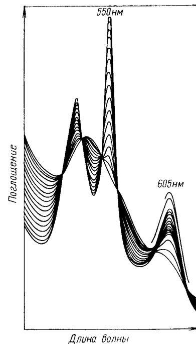
Рис. 3.36. Спектрокулометрическое титрование цитохрома c (17,5 мкмоль/л) и цитохромом c оксидазы (12,5 мкмоль/л) путем восстановления катион-радикалов 1,1'-диметил-4,4'-бипиридила
