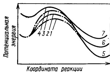
Рис. 14.2. Зависимость потенциальной энергии от координаты реакции превращения адсорбированных (кривые 1—3) и «свободных» радикалов (кривая 4) в продукты электросинтеза Кольбе (кривые 5—7), соответствующие диэкваториальному, диаксиальному или аксиально-экваториальному изомеру)
