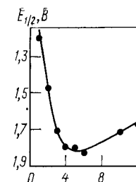
Рис. 12.2. Зависимость потенциалов полуволны бис-(фосфониевых) солей Ph_3P(CH_2)_nPPh_3Br_2 от числа метиленовых групп n в их молекулах
