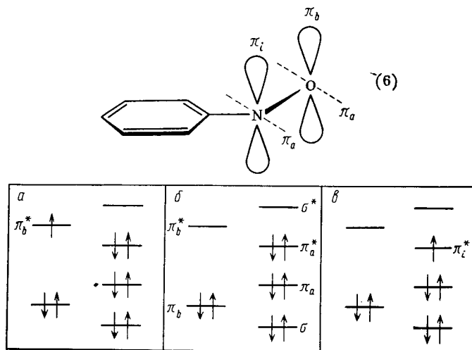
Рис. 2.29. Электронная структура группы NO в анион-радикале (а), нейтральной молекуле (б) и катион-радикале (в) нитробензола
