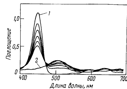
Рис. 3.37. Спектры, полученные с интервалами 0,9 с в ходе восстановления порфирина в 1 М HCl [178]: 1 — субстрат; 2 — продукт реакции
