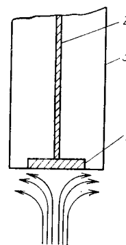
Рис. 3.20. Вращающийся дисковый электрод:
