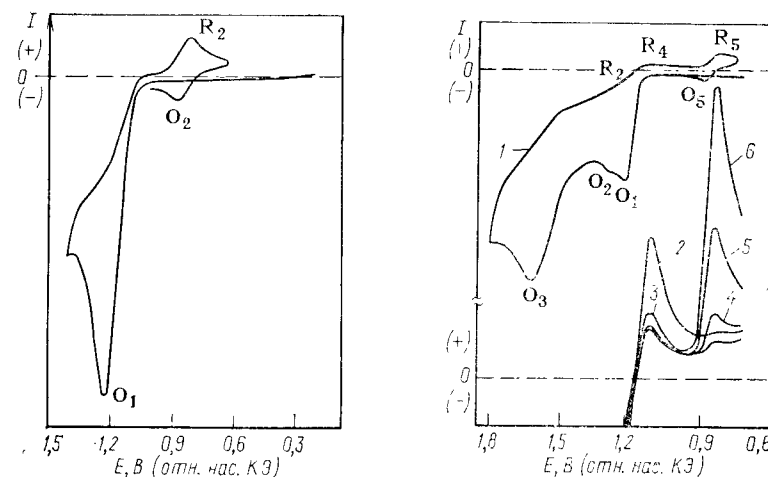
Рис. 3.4. Циклическая вольтамперограмма окисления 1,2-бис(3,4-диметоксифенил)этана (4) в ацетонитриле, содержащем \text{NaClO}_4 (0,1 моль/л) [64] Скорость развертки потенциала 86 мВ/с
