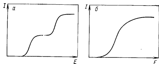
Рис. 2.17. Кривые ток — потенциал, соответствующие восстановлению ароматического углеводорода в неводном апротонном растворителе (а) и в водно-органической среде (б)
