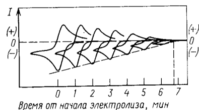
Рис. 3.32. Кривые ток — время в методе кулонометрии при постоянном токе (50 мА) для 2,3,5,6-тетрафенил-1,4-дитиона (0,1 ммоль/л) после окисления в течение 0, 1, 2, 3, 4, 5 и 6 мин (кривые 1—7 соответственно)
