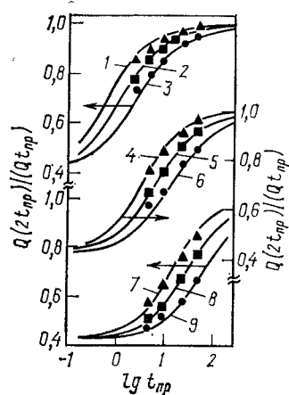
Рис. 3.10. Рабочие кривые в методе хронокулонометрии с двойным ступенчатым изменением потенциала при восстановительной циклизации этилового эфира коричной кислоты:
