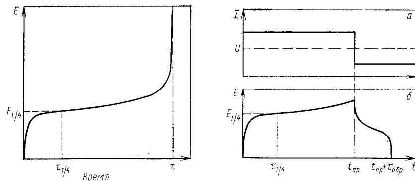
Рис. 3.11. Кривая потенциал — время в методе хронопотенциометрии после наложения постоянного тока
