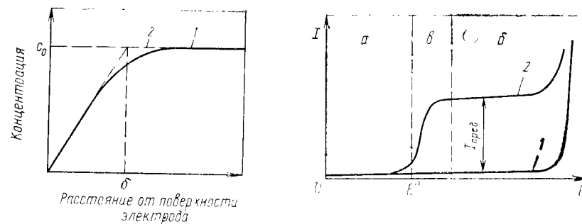
Рис. 3.22. Профиль концентрации вблизи поверхности электрода, когда скорость реакции лимитируется скоростью массопереноса:
