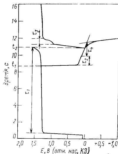
Рис. 3.14. Хронопотенциометрические кривые на платиновом электроде в присутствии тиоксантена (2 ммоль/л) в ацетонитриле на фоне 0,01 моль/л Et_4NClO_4
