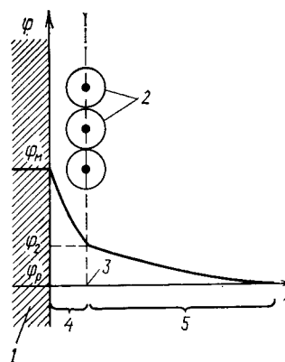
Рис. 2.20. Модель двойного слоя и зависимость потенциала \phi от расстояния x до поверхности электрода в отсутствие специфической адсорбции (молекулы растворителя не показаны):
