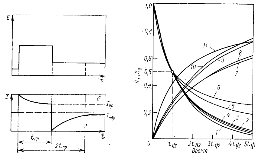
Рис. 3.8. Программа потенциал — время (а) и отклик ток — время (б) при хроноамперометрии с двойным ступенчатым наложением потенциала
