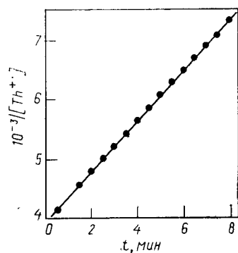
Рис. 3.29. График, подтверждающий второй порядок реакции катион-радикала тиантрена с аннизолом в смеси \text{CH}_2\text{Cl}_2\text{—CF}_3\text{CO}_2\text{H—}(\text{CF}_3\text{CO})_2\text{O} (97 : 2 : 1) [154]
