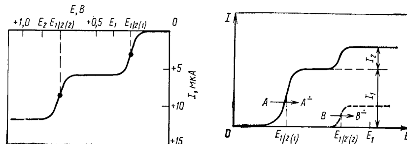
Рис. 2.7. Полная кривая ток — потенциал для фенотиазина (1) [3] Условия эксперимента те же, что приведены на рис. 2.4
