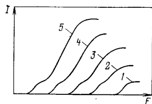
Рис. 2.27. Кривые ток — потенциал для восстановления красителя метиленового голубого на ртутном каплюющем электроде (водная среда, pH 7,96) при концентрациях раствора красителя (в моль/л) [71], равных 0,61 (1), 1,18 \cdot 10^{-4} (2), 2,79 \cdot 10^{-4} (3), 3,67 \cdot 10^{-4} (4), 4,54 \cdot 10^{-4} (5) моль/л. Для наглядности кривые сдвинуты по оси потенциалов.
