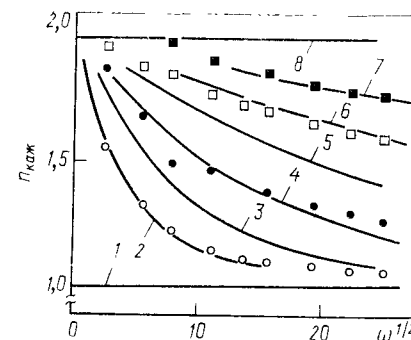
Рис. 3.24. Рабочие кривые для механизма ECE при значениях константы скорости (в \text{с}^{-1} ) стадии C , равных 0 (1), 3 (2), 10 (3), 30 (4), 100 (5), 300 (6), 1000 (7), \infty (8)
