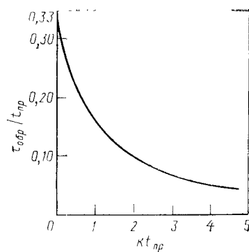
Рис. 3.13. Рабочая кривая в методе хронопотенциометрии с обращением тока для процесса EC [95]
