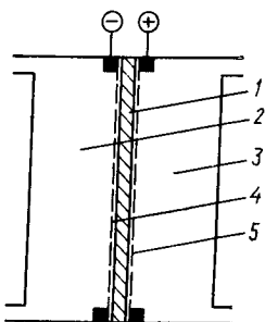
Рис. 5.10. Ячейка с сетчатыми электродами, прижатыми с двух сторон к твердому полieleктролиту [17]: 1 — ионообменная мембрана; 2, 3 — катодное и анодное пространства соответственно; 4 — катод; 5 — анод
