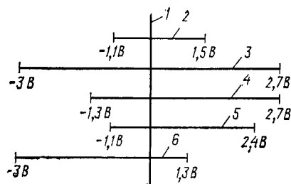
Рис. 2.11. Области электроактивности для нескольких растворов, содержащих \text{Et}_4\text{NClO}_4 ( 10^{-1} моль/л), на платиновом электроде (потенциалы приведены относительно каломельного электрода в водной среде):
