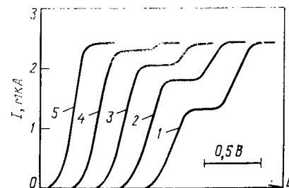
Рис. 3.18. Влияние увеличивающейся активности протонов ( 1 < 2 < 3 < 4 < 5 ) на вид полярограмм антрацена
