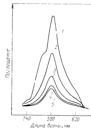
Рис. 3.38. Спектры поглощения анион-радикала перилена в ДМФА, содержащем уксусную кислоту (70 ммоль/л), измеренные методом модуляции зеркального отражения при 3 (1), 10 (2), 30 (3), 60 (4) и 80 (5) Гц [179]
