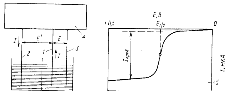
Рис. 2.3. Трехэлектродная ячейка для измерения кривых ток — потенциал: 1 — рабочий (индикаторный) электрод; 2 — вспомогательный электрод (противоэлектрод); 3 — электрод сравнения; 4 — потенциостат
