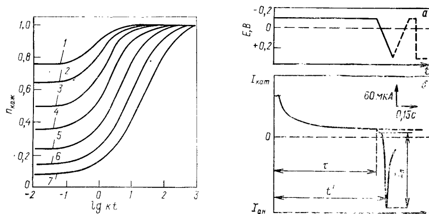
Рис. 3.6. Рабочие кривые для процесса ЕС в методе хроноамперометрии при различных потенциалах (в В) [76]:
