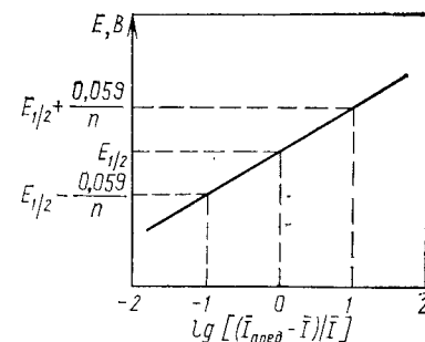
Рис. 3.16. Полярграмма в случае обратимой реакции \text{Ox} + ne \rightleftharpoons \text{Red} ( I_{\text{пред}} отсчитывается от полярграммы фона)
