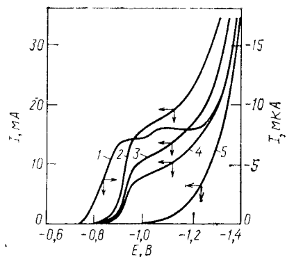
Рис. 4.1. Вольтамперные кривые 4-цианоацетофенона, полученные на ртутном каплюющем (1) и перемешиваемом ртутном донном (2—5) электродах (0,15 М \text{H}_2\text{SO}_4 ; 1 \cdot 10^{-3} моль/л деполаризатора):
