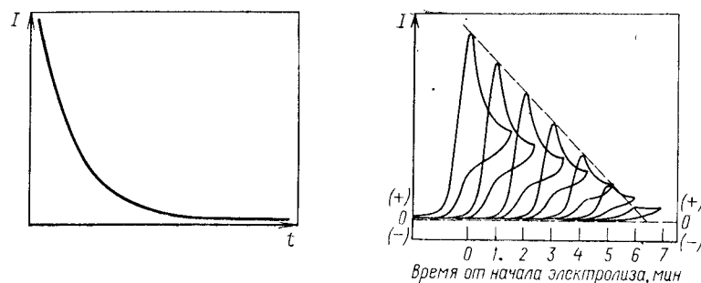
Рис. 3.30. Зависимость тока I от времени t при электролизе при постоянном потенциале (кулонометрия)
