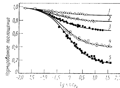
Рис. 3.39. Рабочие кривые для механизма ECE_{\text{гом}} в методе хроноабсорбметрии [184]
