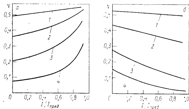
Рис. 3.28. Зависимость коэффициента эффективности N от отношения I/I_{\text{пред}} на вращающемся дисковом электроде при различных значениях безразмерного параметра ХКТС (кривые 1—4; подробнее см [130, 133]) для различных механизмов димеризации:
