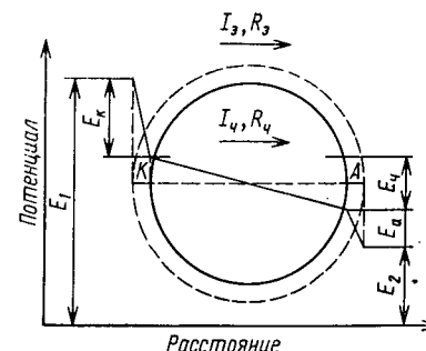
Рис. 5.12. Распределение потенциала в биполярной частице [74]: A, K — анодная и катодная зоны соответственно; I_3, R_3 — ток и сопротивление электролита; I_4, R_4 — ток и сопротивление частицы; E_1 и E_2 — потенциалы в электролите; E_A, E_K — анодный и катодный потенциалы; E_Ч — омическое падение напряжения в частице
