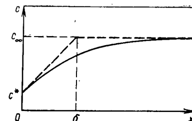
Рис. 2.12. Зависимость концентрации частиц, восстанавливающихся на плоском электроде, от расстояния до электрода (пунктирной линией показана зависимость, соответствующая эмпирическому приближению Нернста)
