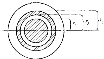
Рис. 3.25. Схематическое изображение вращающегося дискового электрода с кольцом
