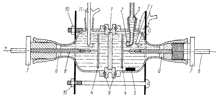
Рис. 5.4. Ячейка для электролиза:
