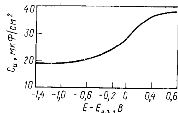
Рис. 2.25. Зависимость интегральной емкости C_{н.} от потенциала для ртутного электрода в 0,5 М водном растворе \text{Na}_2\text{SO}_4
