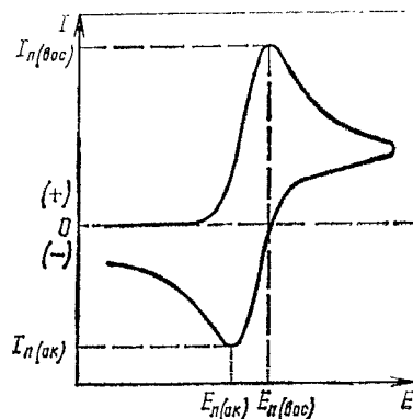
Рис. 3.3. Циклическая вольтамперограмма нернстовской системы
