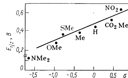
Рис. 2.30. Зависимость потенциалов полуволны E_{1/2} некоторых пара-замещенных N -антралианилинов от констант \sigma^+ :
