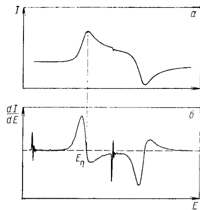
Рис. 3.2. Циклические вольтамперограммы:
