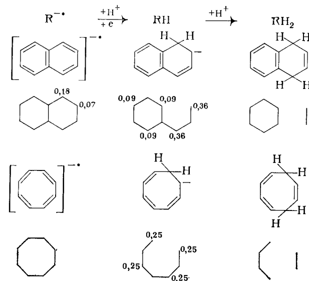
Рис. 6.1. Заряды, рассчитанные методом МОХ, для продуктов электровосстановления нафталина и циклооктатетраена:
