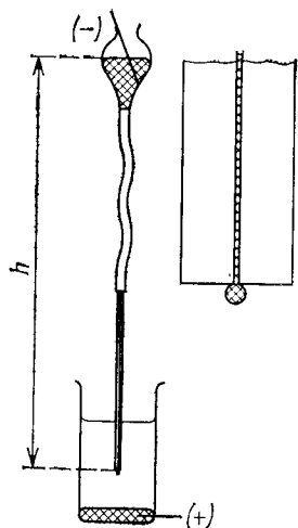
Рис. 3.15. Схематическое изображение ртутного капающего электрода
