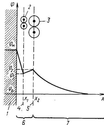
Рис. 2.22. Модель двойного слоя и зависимость потенциала от расстояния до поверхности электрода в случае специфической адсорбции аниона [42]:
