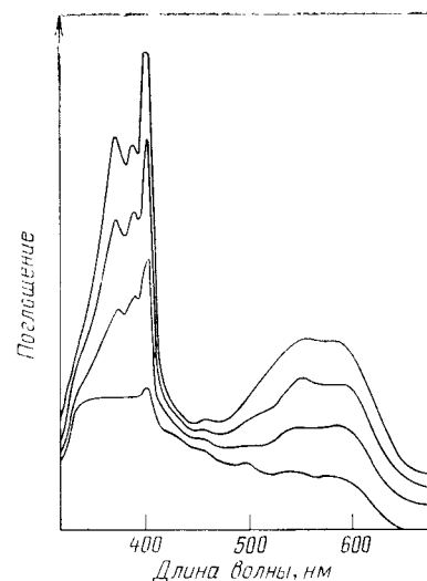
Рис. 3.35. Спектры катион-радикала 1,1'-дибензил-4,4'-бипиридила, полученные через равные промежутки времени восстановления соответствующего дикатиона на оптически прозрачном катоде из \text{SnO}_2 [173]
