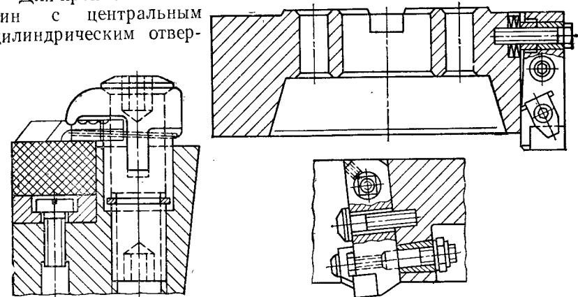
Рис. 2.34. Сборная торцовая фреза с регулируемыми вставками с пластинами из керамики фирмы «Фельдмюлле»
