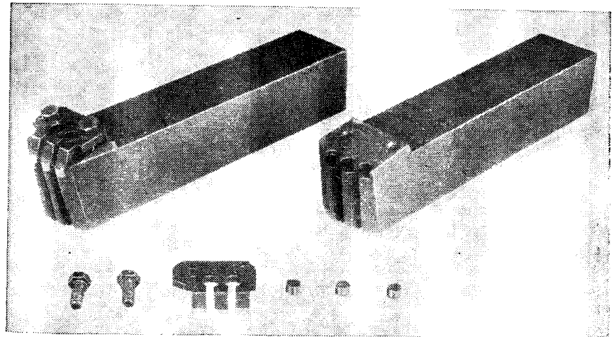
Рис. 2.9. Резец токарный ступенчатый для обработки прокатных валков
