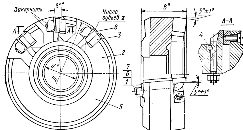
Рис. 2.24. Фреза торцовая с механическим креплением квадратных пластин из керамики:
