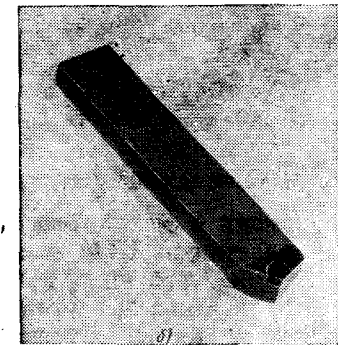
Рис. 2.3. Расточные резцы, оснащенные композитом 01 или 10: а — конструкция; 1 — круглого сечения; 2 — прямоугольного сечения; б — общий вид
