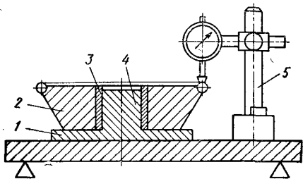
Рис. 2.12. Приспособление для настройки торцового биения ножей регулируемой фрезы вне станка: 1 — опорный фланец; 2 — фреза; 3 — сменная центрирующая втулка; 4 — штифт; 5 — магнитная стойка с микроиндикатором
