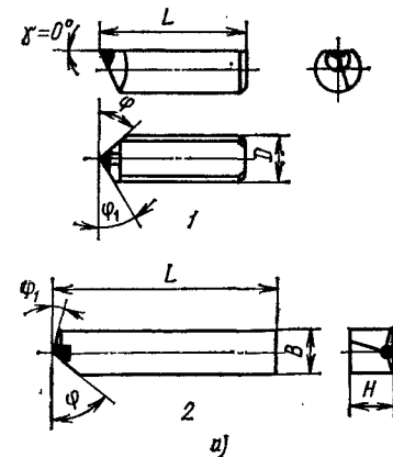
Рис. 2.3. Расточные резцы, оснащенные композитом 01 или 10: а — конструкция; 1 — круглого сечения; 2 — прямоугольного сечения; б — общий вид
