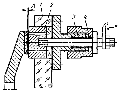
Рис. 5.3. Конструкция катода, обеспечивающего работу алмазного круга на металлической связке в режиме самозаточивания
