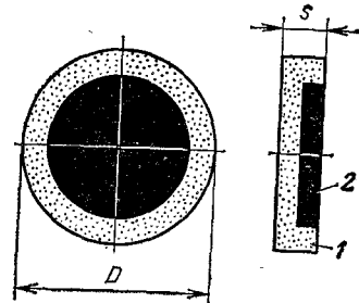
Рис. 2.18. Двухслойные заготовки для напайного инструмента: 1 — твердый сплав; 2 — алмазный рабочий слой
