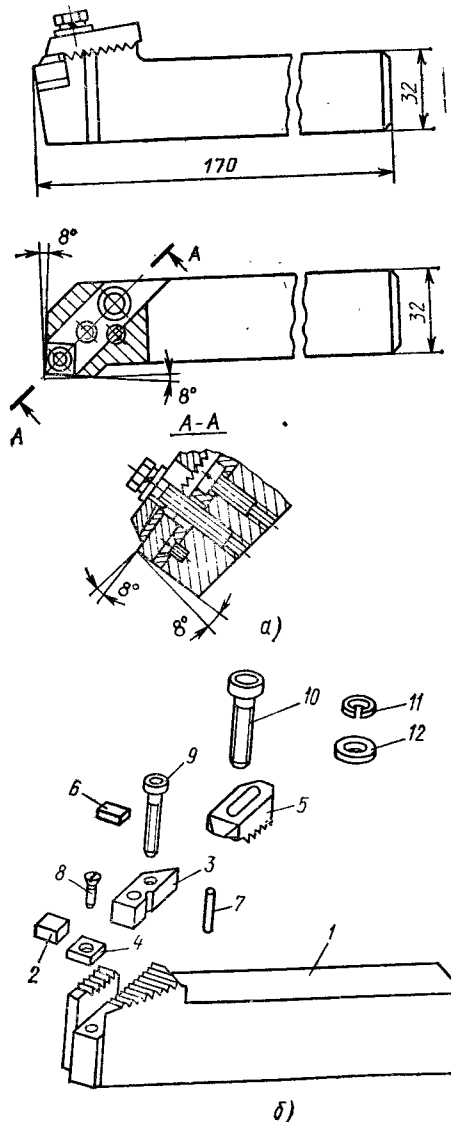
Рис. 2.25. Специальный токарный резец с пластинами из керамики: а — конструкция; б — конструктивные элементы
