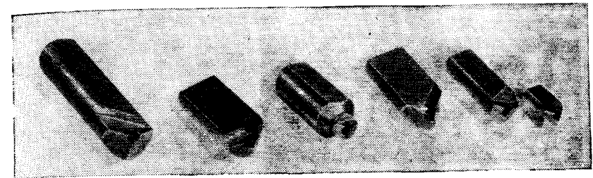
Рис. 2.1. Вставки режцовые с неразъемно закрепленным (запаянным) поликристаллом композитов 01, 02 или 10
