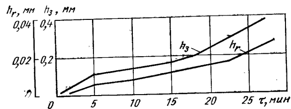
Рис. 3.3. Зависимость радиального износа h_r и износа по задней поверхности h_3 от продолжительности обработки \tau резцами с пластинами из керамики В-3: v = 150 м/мин; S_0 = 0,15 мм/об; t = 0,3 мм
