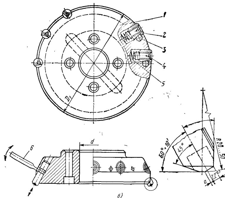
Рис. 2.11. Фреза торцовая насадная регулируемая со вставными перетачиваемыми ножами, оснащенными композитами 01 или 10:
