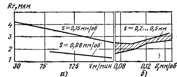
Рис. 3.2. Влияние скорости резания v при t = 0,5 мм (а) и подаче S_0 при v = 150 м/мин (б) на параметр шероховатости обработанной поверхности Rz
