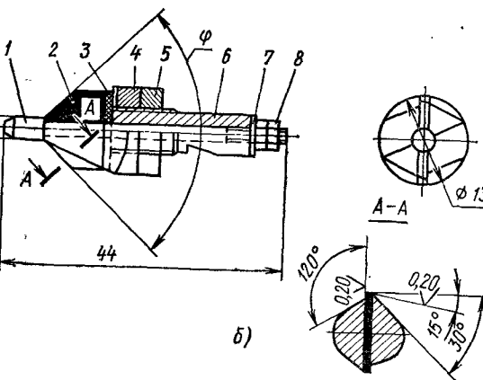
Рис. 2.17. Зенковка с механическим креплением пластин из композита 05: а — общий вид; б — конструкция d = 3 \dots 6 мм; \Phi равно 90° и 120°; 1 — направляющий штырь; 2 — специальная пятигранная перетачиваемая пластина из композита 05; 3 — демпфирующая шайба; 4 — корпус; 5 — контргайка; 6 — полый винт-хвостовик; 7 — шайба; 8 — гайка
