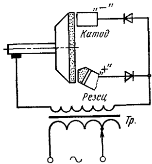
Рис. 5.2. Принципиальная схема модернизации универсально-заточного станка, обеспечивающей одновременную правку круга и разупрочнение обрабатываемой поверхности резца
