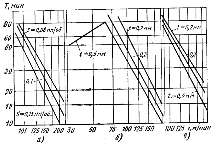
Рис. 3.1. Зависимость стойкости T резцов из керамики В-3 от скорости резания при t = 0,3 мм (а), S_0 = 0,15 мм/об (б), S_0 = 0,08 мм/об (в)
