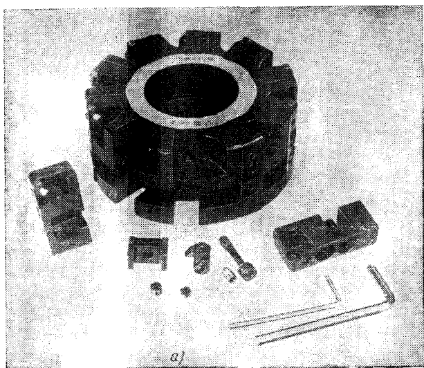
Рис. 2.13. Фреза торцовая насадная регулируемая кассетной конструкции с механическим креплением неперетачиваемых прецизионных пластин из композитов 01, 05, 10Д: а — общий вид; б — конструкция (см. стр. 41)
