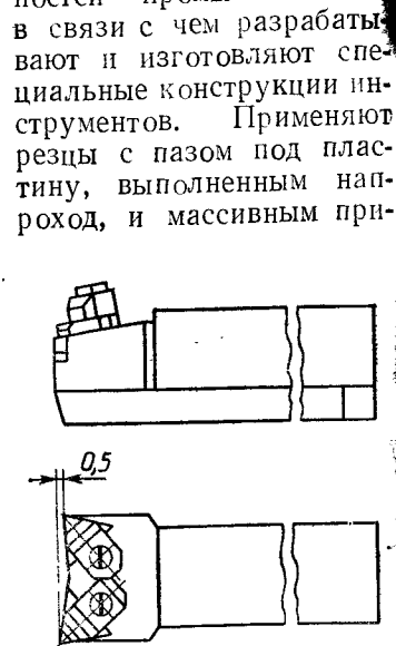
Рис. 2.26. Двусторонний токарный резец с пластинами из керамики для наружного точения и растачивания
