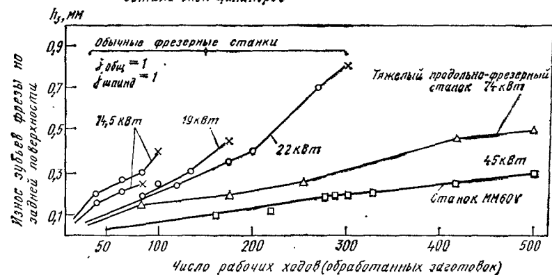
Рис. 6.1. Зависимость износа торцевой фрезы диаметром 300 мм, z = 24 с пластинами из оксидно-карбидной керамики от жесткости фрезерного станка J при обработке плоскости блока цилиндров двигателя из чугуна с v = 400 м/мин ( n = 400 мин -1 ; S_z = 0,26 мм/зуб; S_M = 2000 мм/мин, t = 0,5 мм (для тяжелого продольно-фрезерного станка J_{общ} = 2 , J_{шпинд} = 2,75 , для станка ММ60V J_{общ} = 4 , J_{шпинд} = 3 ))
