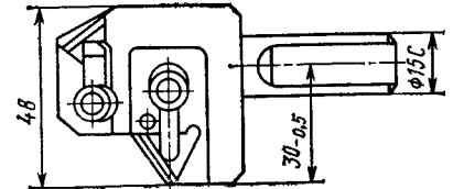
Рис. 2.29. Расточная оправка с пластинами из керамики для станков с ЧПУ
