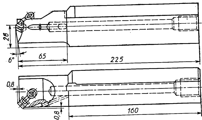
Рис. 2.32. Специальный резец с механическим креплением пластин из керамики с подводом СОЖ
