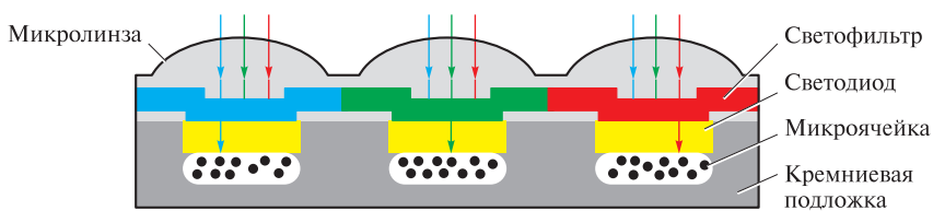
Рис. 25.2. Схематичное изображение фрагмента CCD-матрицы
