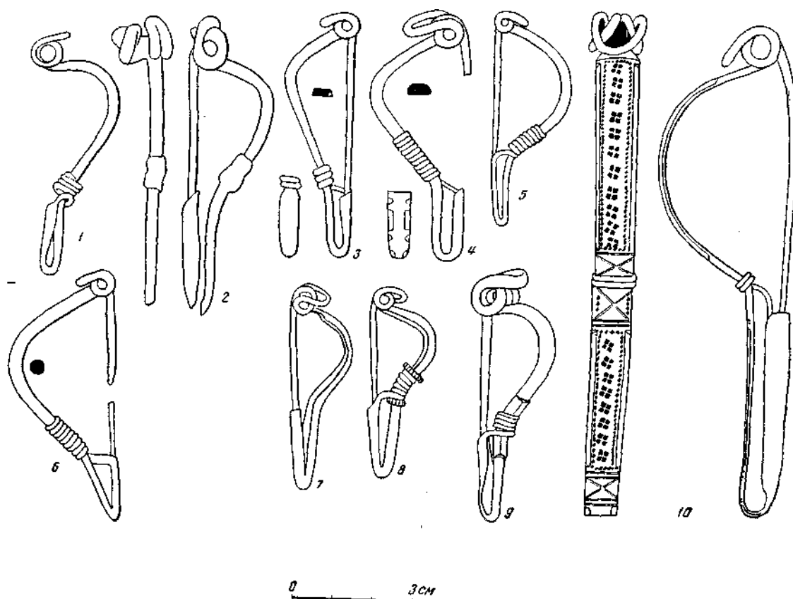
Рис. 3. Одночленные прогнутые подвязные фибулы с узкой ножкой Среднеевропейская серия (стр. 58—59): первый вариант — 1, 2, второй вариант — 3—9, третий вариант — 10
