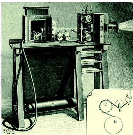
Проекционный аппарат «Хром», который использовал Леон Гомон.
